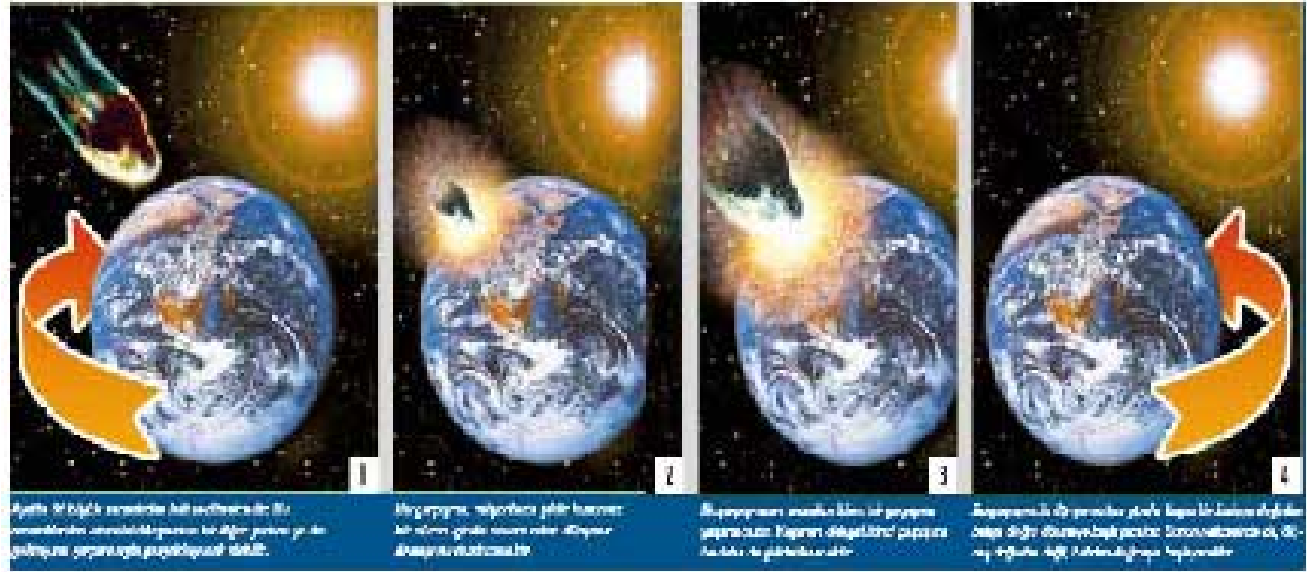
Şekil -3 Birinci olayın temsili resmi: Dünyanın başka bir Güneşle çarpışması.
