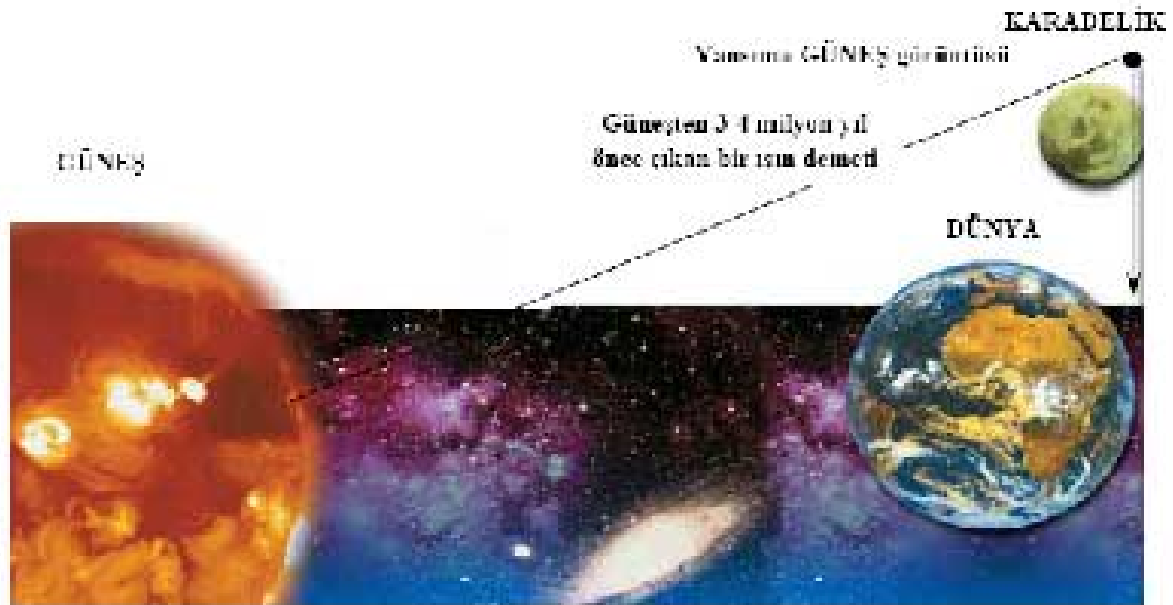
Şekil -4 İkinci olayın temsili resmi: Güneşten çıkan bir ışının bir Karadelikten yansması.
