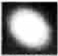
VIRGO
